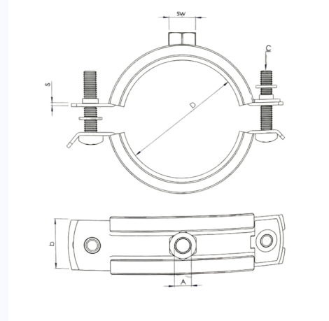
Teknik Çizim / Technical Drawing
